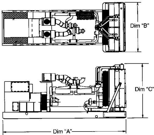
标准机组示意图
